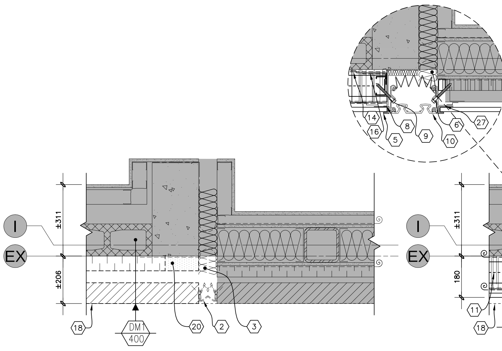
8 VUE EN PLAN TYPE 051,101 452 1:10mm
