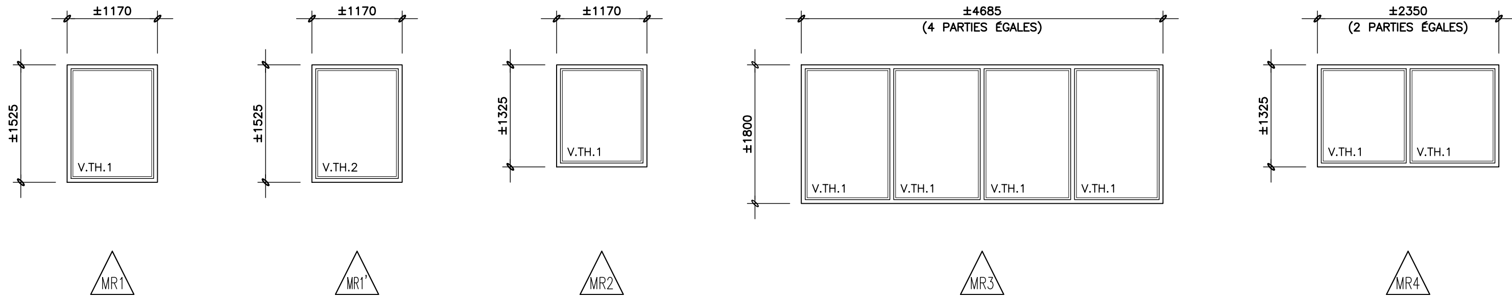
ÉLÉVATIONS TYPES DES MURS RIDEAUX 1:50mm (VUE DE L'EXTÉRIEUR)
