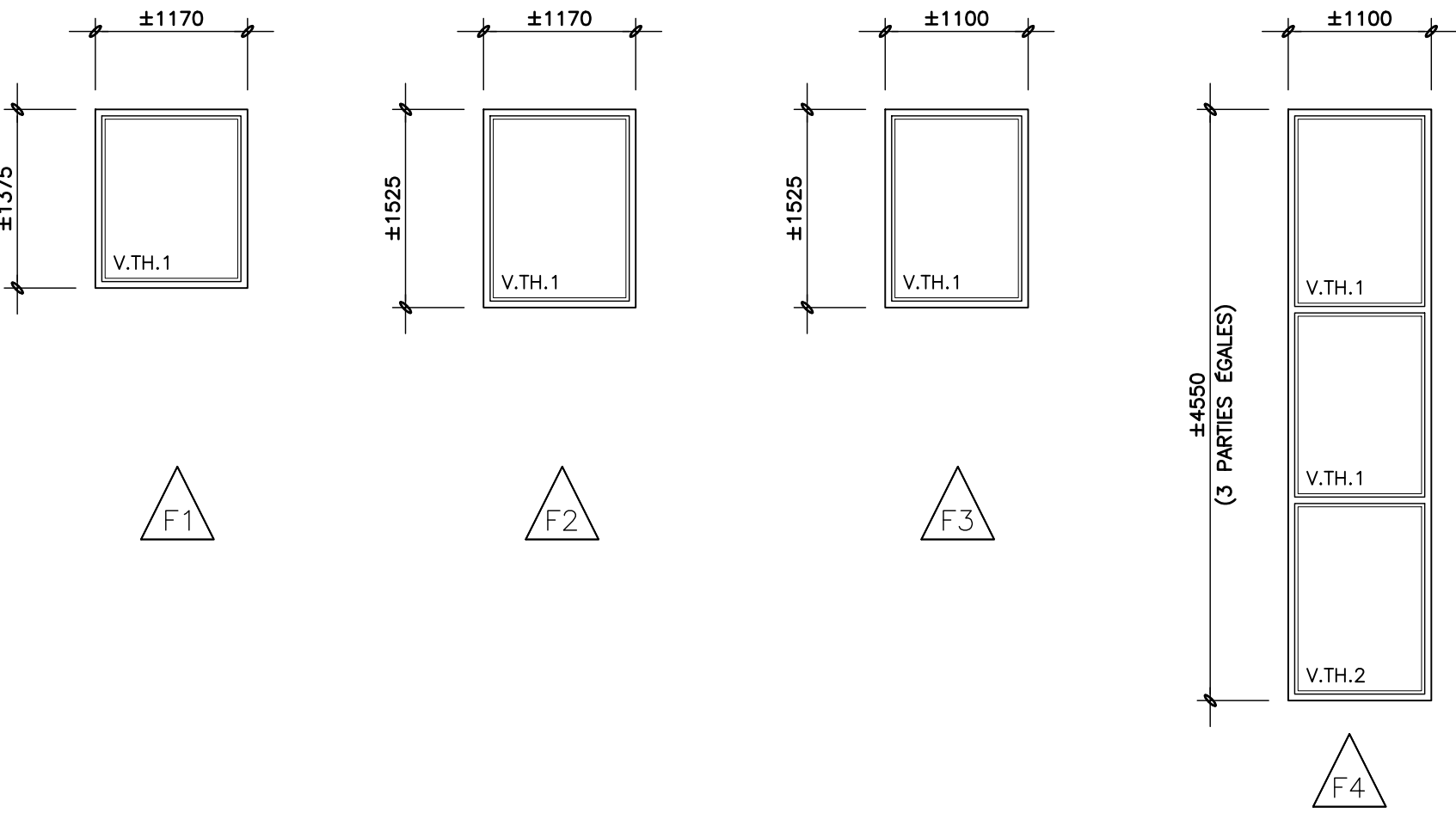
ÉLÉVATIONS TYPES DES FENÊTRES 1:50mm (VUE DE L'EXTÉRIEUR)
